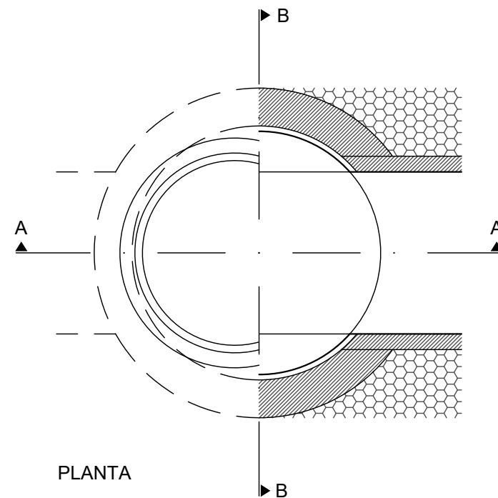
POU DE REGISTRE PER A SANEJAMENT
