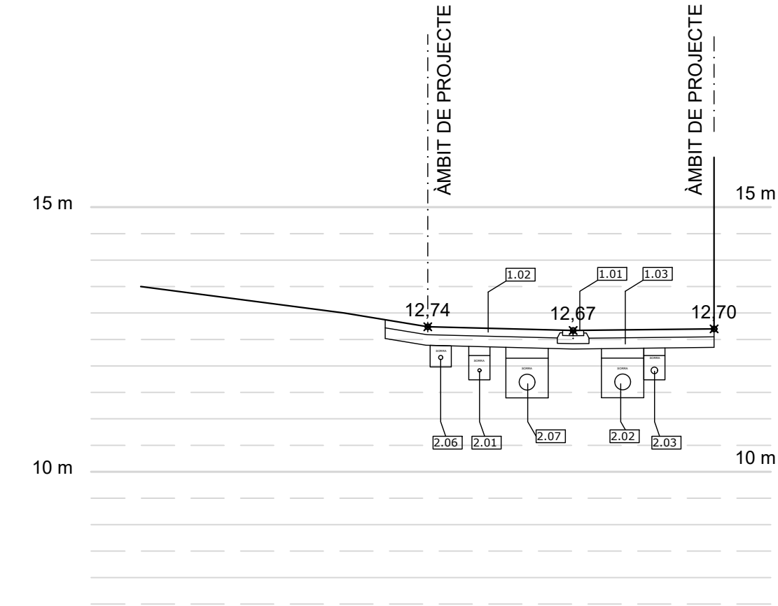
SECCIÓ TRANSVERSAL ST1 PROJECTADA E:1/100
