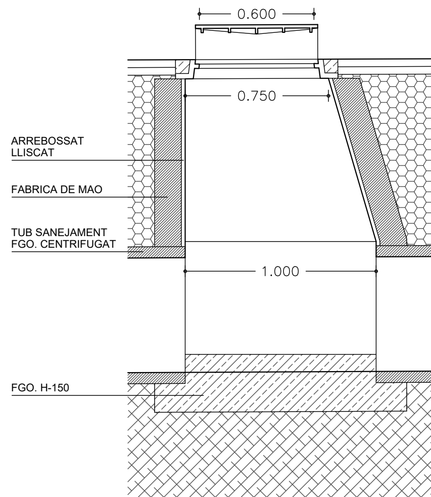
SECCIO A-A
