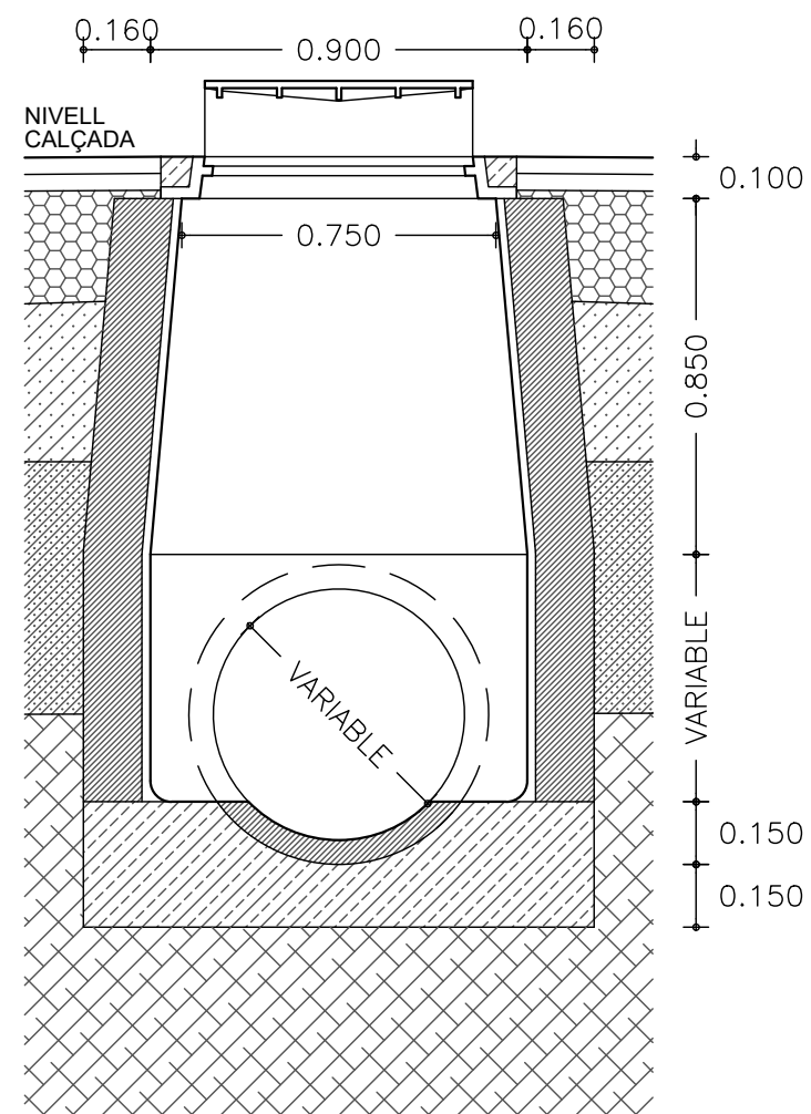
SECCIO B-B
