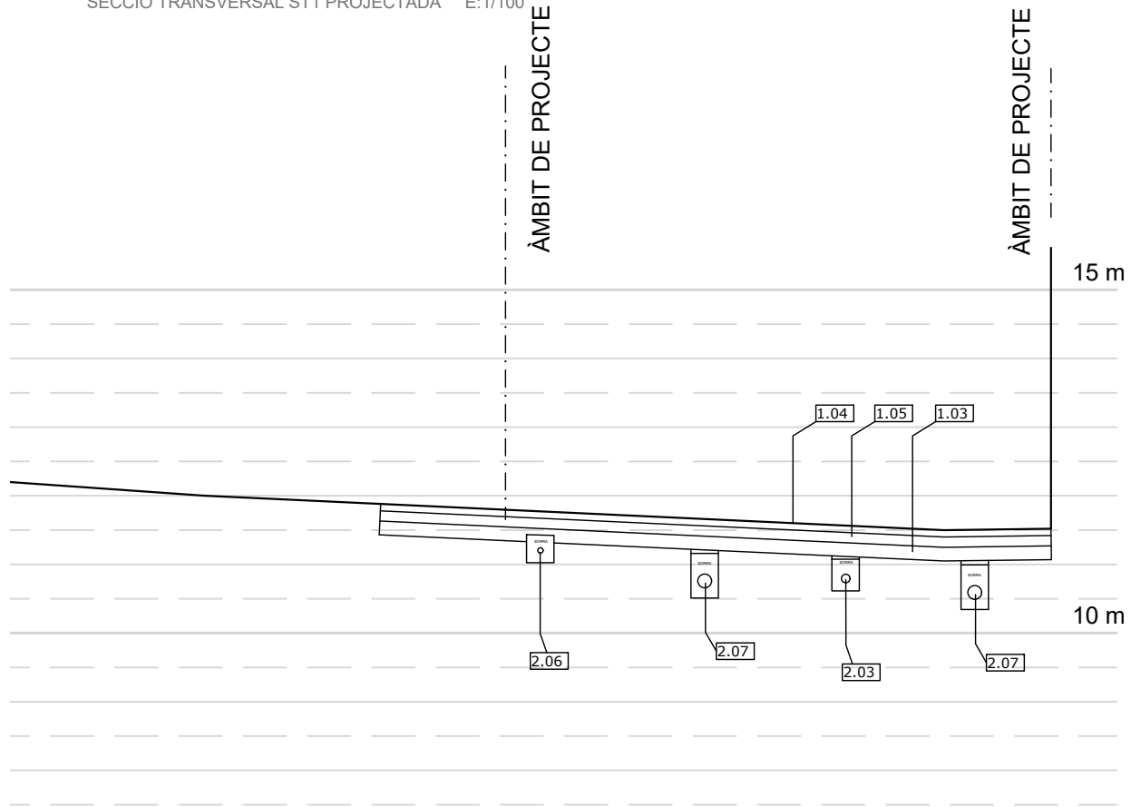
SECCIÓ TRANSVERSAL ST1 PROJECTADA E:1/100
