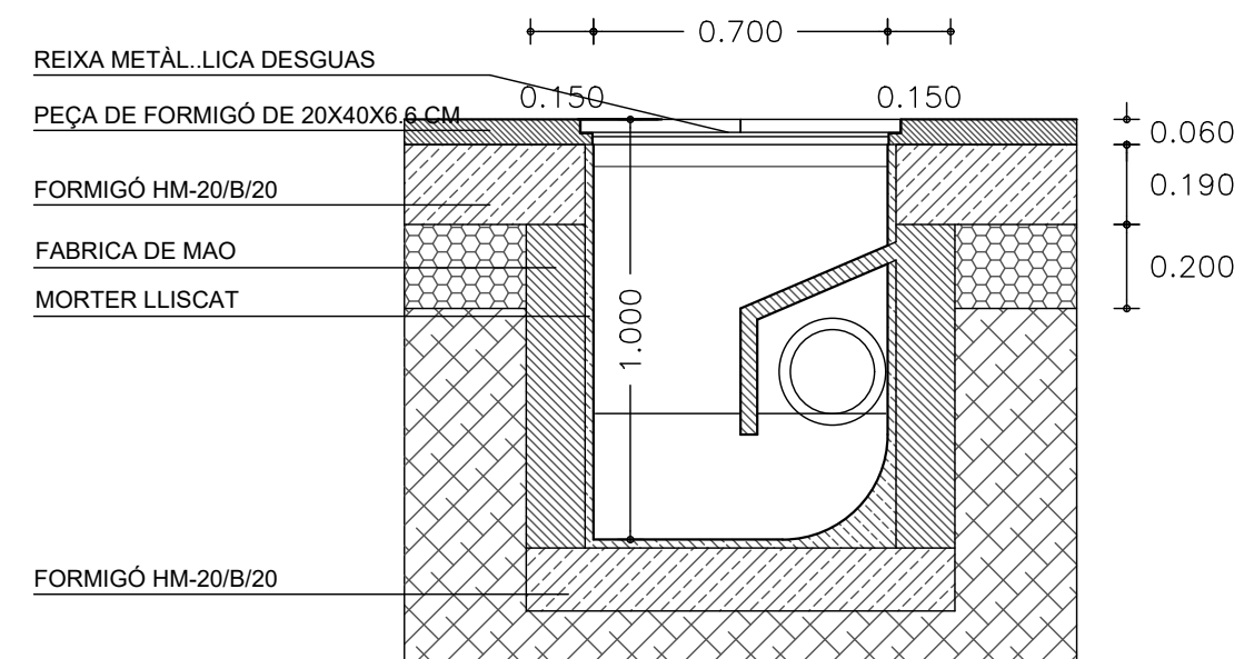
SECCIO A-A
