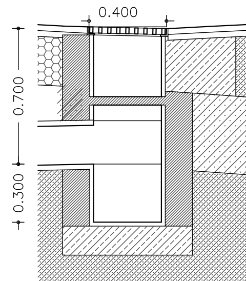
SECCIO B-B
