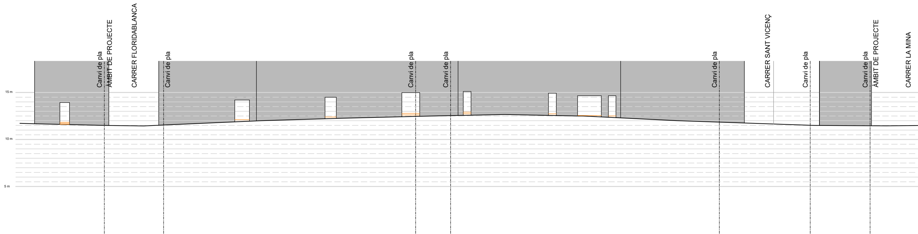
SECCIÓ LONGITUDINAL PROJECTADA E:1/200
